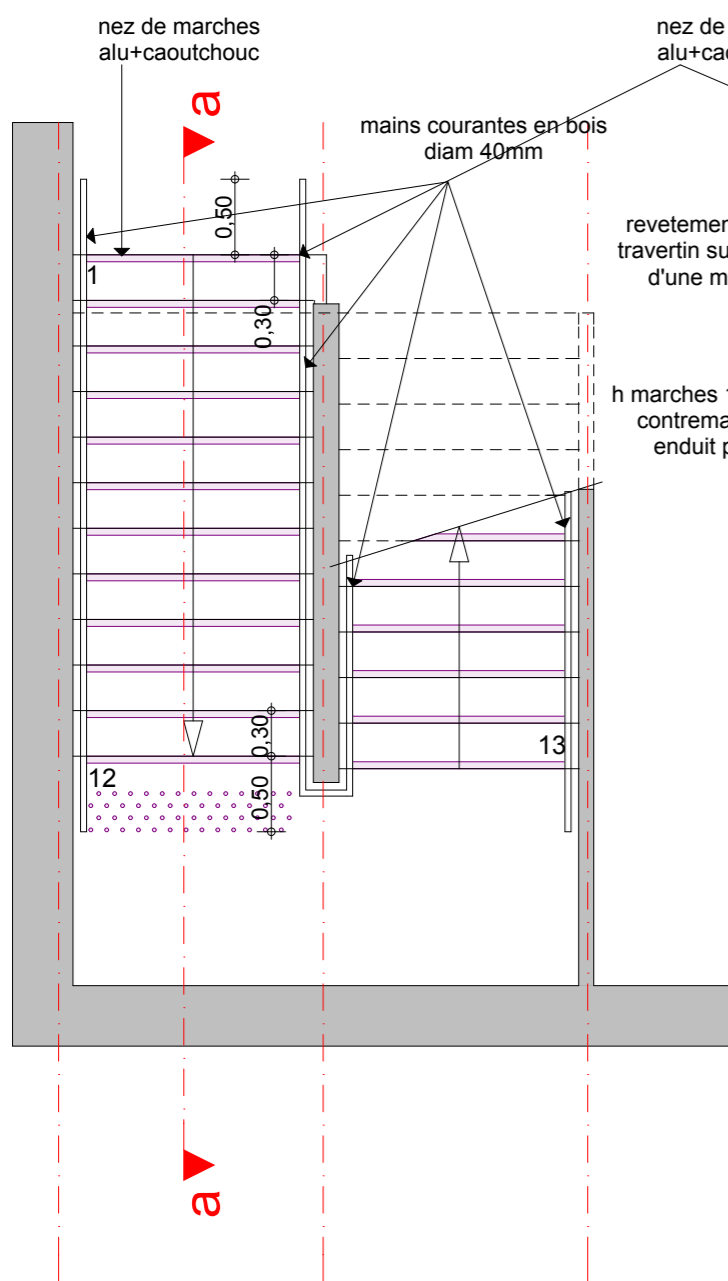
plan RDC
